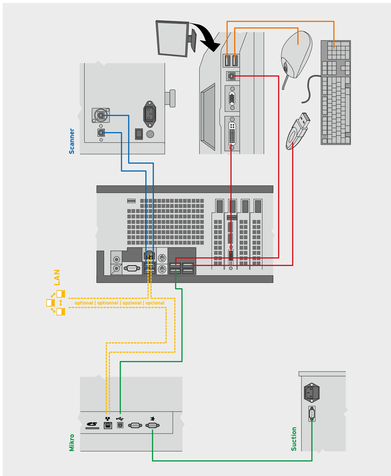
Connection diagram milling machine Schéma de raccordement de l'appareil de fraisage Schema di collegamento fresatore Diagrama de conexiones para fresadora
